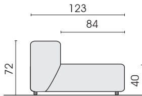
Seitenansicht
